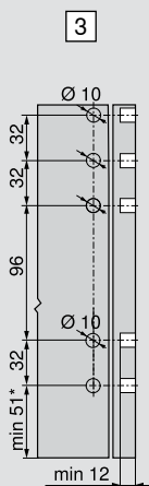
Wymiary nawierć frontu w wersji EXPANDO
