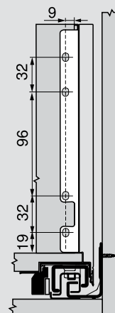
Wymiary montażu ścianki tylnej
