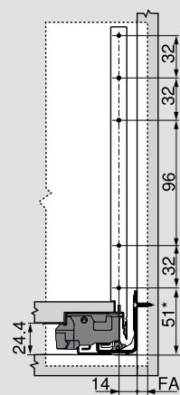
Wymiary montażu frontu w wersji na wkręty
