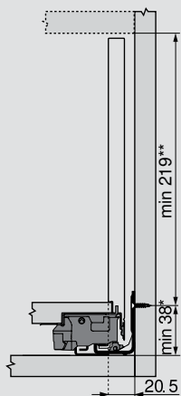
Wymiary zabudowy w korpusie
