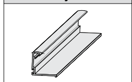
Profil ramkowy L24 Slim Line
