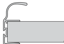
Sposób montażu rączki z płytą # 18 mm
