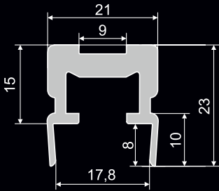
Profil łączący do rury 20×20 Профиль соединительный для трубы 20×20
