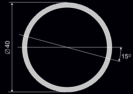
Rura Ø 40 mm do ścianek działowych Труба Ø 40 для офисных перегородок
